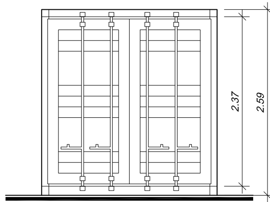
Alçado Frontal
