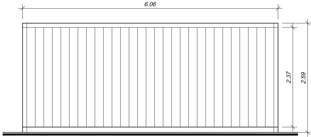
Alçado Lateral
